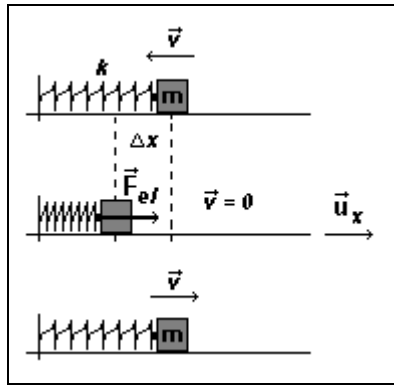
Figura 5.9 – Força elástica de uma mola de constante elástica k , comprimida de \Delta x .
