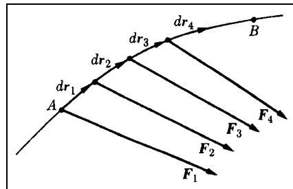
Figura 5.3 – Trabalho total (soma dos inúmeros trabalhos infinitesimais).
