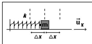
Figura 5.10 – Sistema - mola elástica e massa oscilante.
