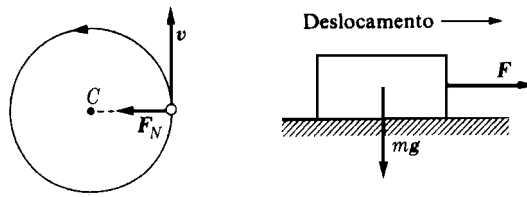
Figura 5.2 – Trabalho (nulo) de uma força perpendicular ao movimento.
