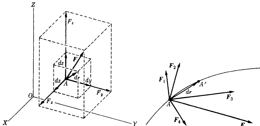
Figura 5.5 – Trabalho total, das componentes ou de várias forças aplicadas.
