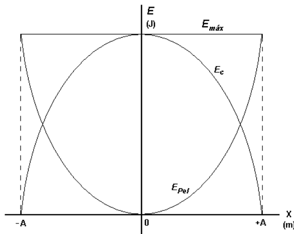
Figura 5.11 – Variação de energia cinética e potencial elástica, num sistema oscilante.
