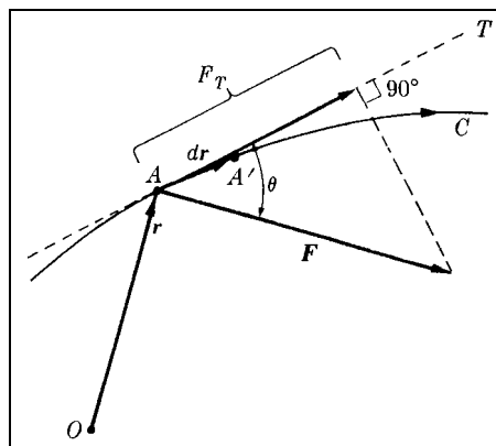
Figura 5.1 – Trabalho elementar de uma força.
