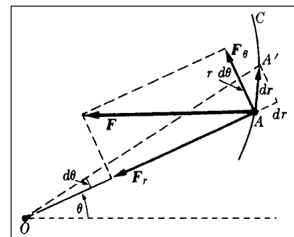
Figura 5.7 – Componentes da Força.
