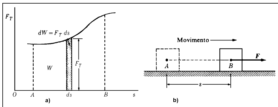
Figura 5.4 – a) Representação da força versus deslocamento. b) Trabalho de uma força constante.
